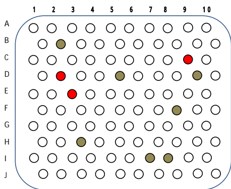
(a)伝熱管配置図および検査結果
